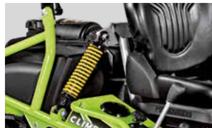
10.27 Système de ressort sur châssis-siège
